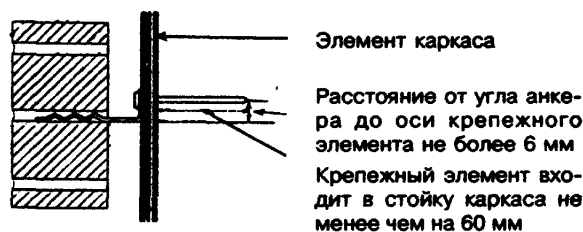
Рисунок 10-1 — Анкеры в каменной облицовке
