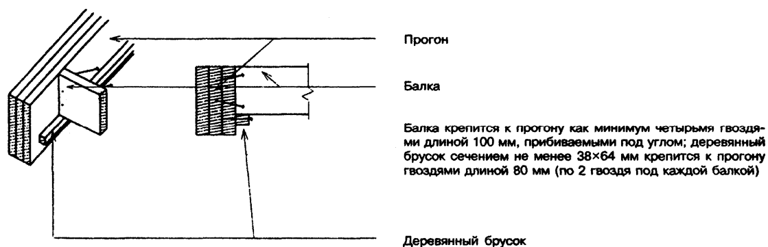
Рисунок 6-8 — Варианты крепления балок перекрытия к боковой поверхности деревянных прогонов
