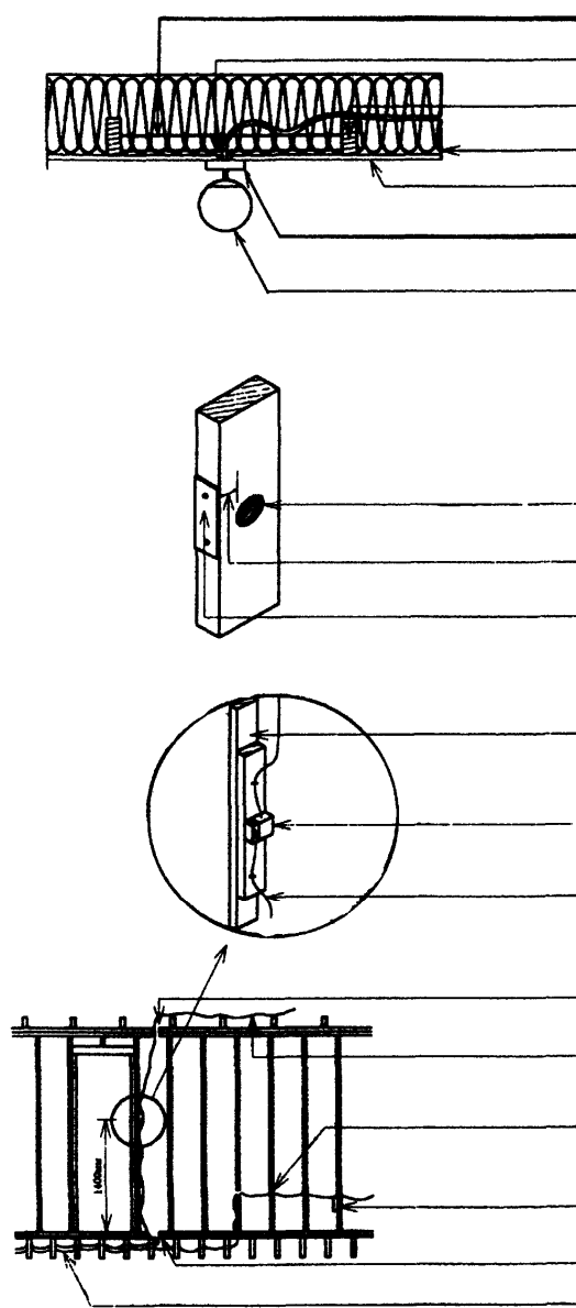
Рисунок 13-9 — Прокладка электрических проводов в элементах каркаса
