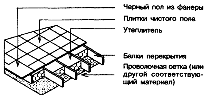
Перекрытие над неотапливаемым подпольем, утепленное насыпным утеплителем
