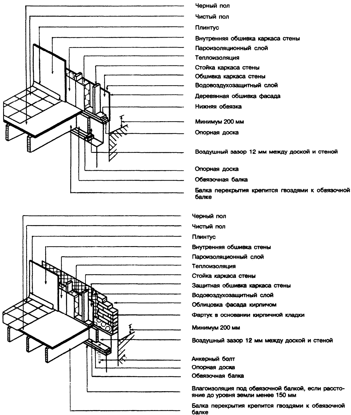
Рисунок 6-5 — Опираие балок перекрытия на опорную доску, уложенную на уступ фундаментной стены
