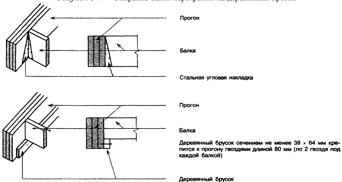
Рисунок 6-7 — Опираие балок перекрытия на деревянный прогон
