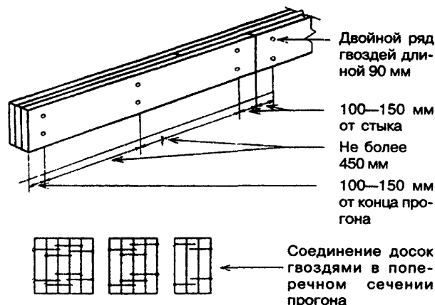
Рисунок 6-1 — Деревянные прогоны составного сечения
