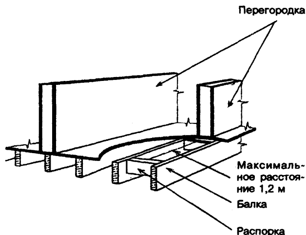
Рисунок 6-13 — Опираение перегородок
