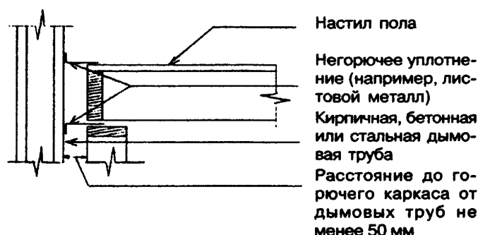
Рисунок 13-3 — Расстояние от дымовой трубы до строительных конструкций
