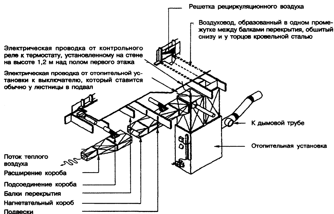
Рисунок 13-4 — Крепление воздуховодов
