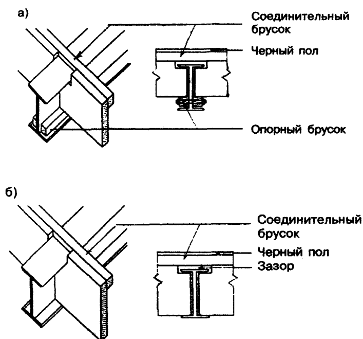
а — балки опираются на деревянные бруски, уложенные на нижние полки прогона; б — балки опираются непосредственно на нижние полки прогона
