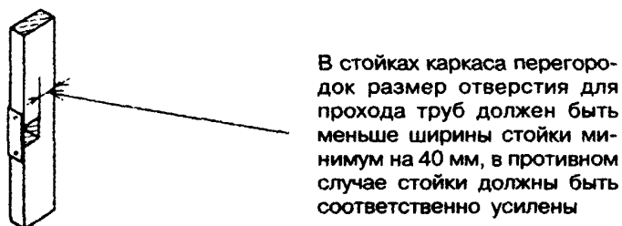
Рисунок 13-7 — Вырезы в стойках каркаса для прохода труб
